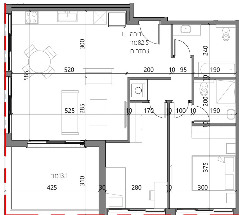
קומה טיפוסית - דירה E 1 : 100
